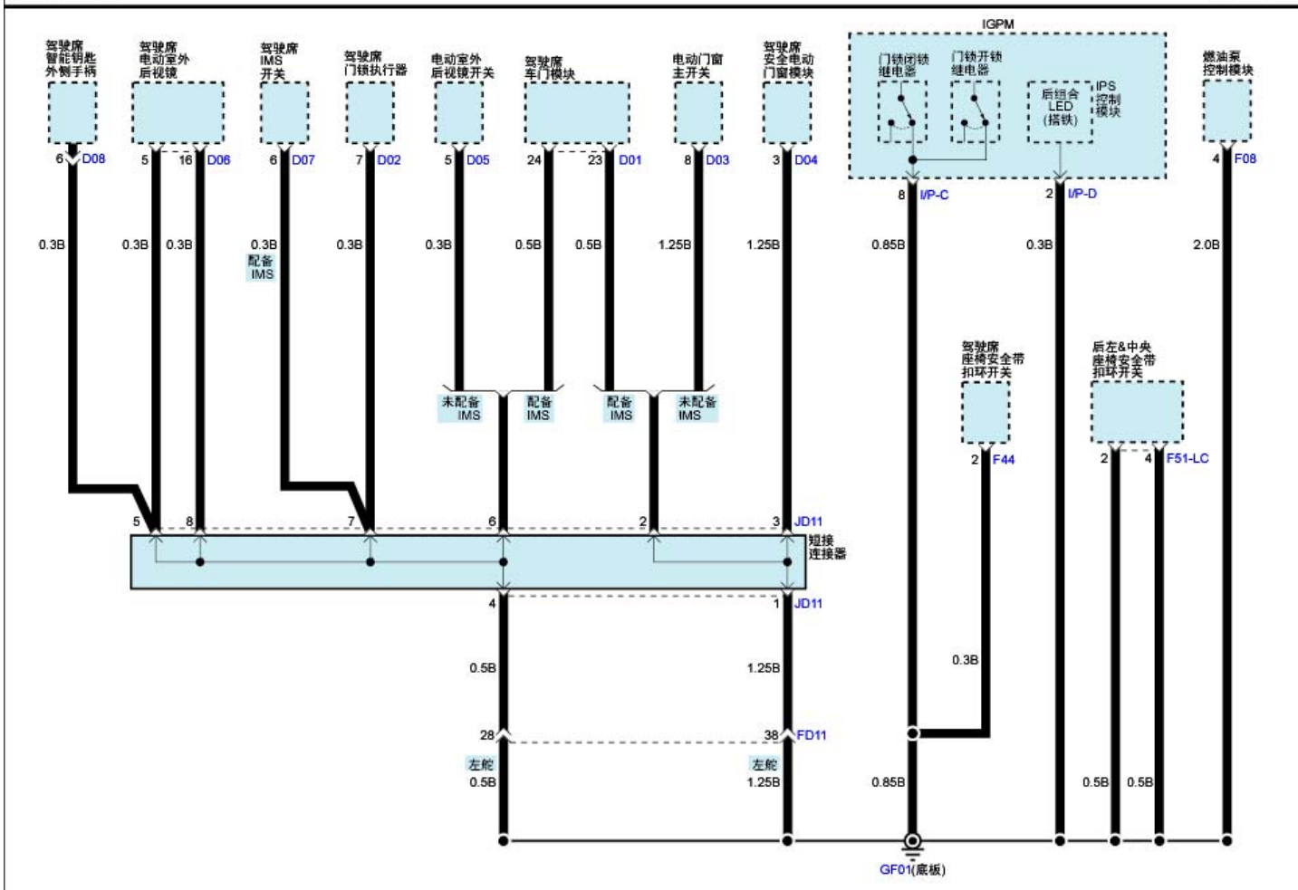
搭铁分布(6)
